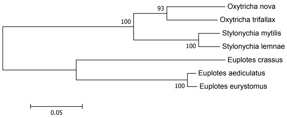
Euplotes Oxytricha Stylonychia telomerase RNA
